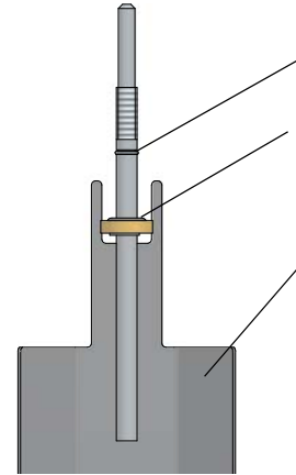
Двойное уплотнение электродов для парового цилиндра CY45/2 (SLE45/65)
